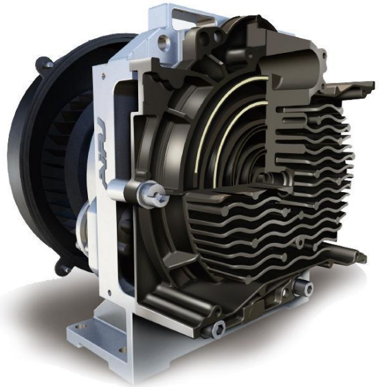
спиральный блок производства AIPU (Китай)
